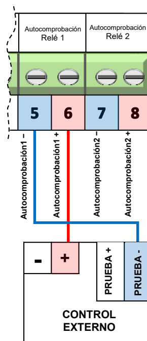
Ejemplo de armario de automatización con autocomprobación negativa (DIP1=ON) en el relé 1
