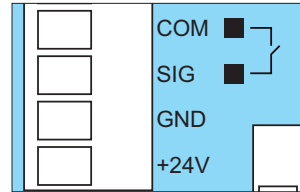
Borne de raccordement pour barrière lumineuse 4 fils
