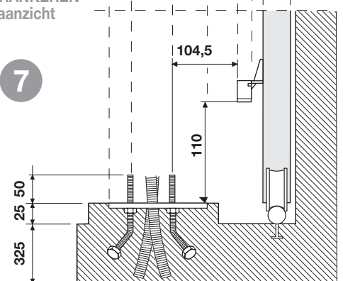
DE MOTOR VERANKEREN Zijaanzicht
