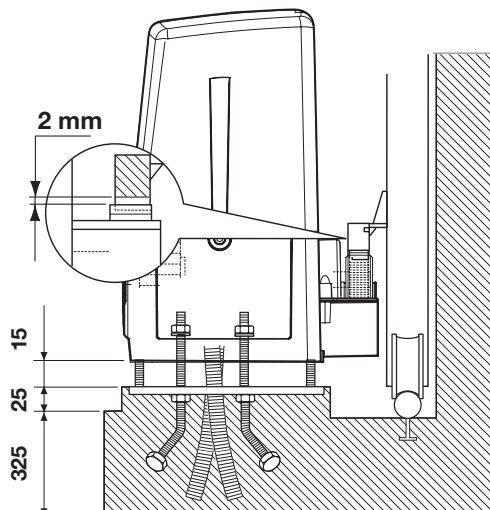
DE MOTOR VERANKEREN Bovenaanzicht
