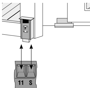
Connexion serrure de verrouillage électrique (12 V-15 W max.)
