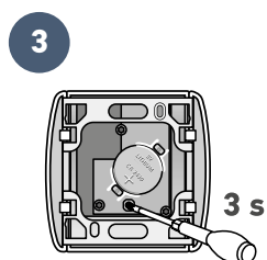
Tyłna część punktu sterowania
